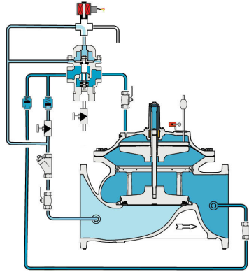
反向水流
