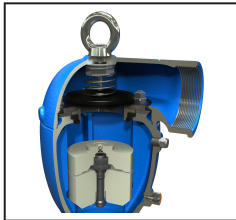
עם מניעת כניסת מים (C70-IP)
