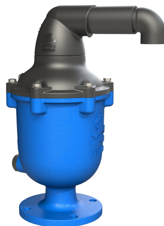
C50-P-带法兰，带浪涌保护和90度弯头
