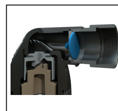
Prevenção de Entrada (código C50-IP)
