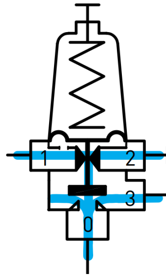
Válvula principal abierta Presión del sistema Mayor que el ajuste: 0 <--> 3 <--> 1
