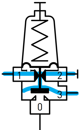
Válvula maestra cerrada Presión del sistema inferior al ajuste: 0 <--> 3 <--> 1
