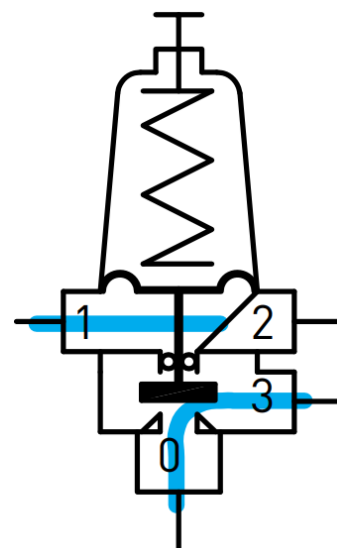
Ouverture modulante Pression régulée supérieure au réglage : 0 < \text{---} > 3''
