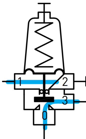
Position stable Pression régulée égale au réglage : 0 < \text{---} > 3 passage contrôlé
