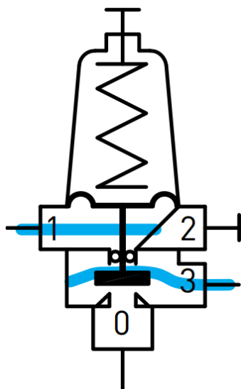
Fermeture modulante Pression régulée Inférieure au réglage : 0 < \text{---} > 3''
