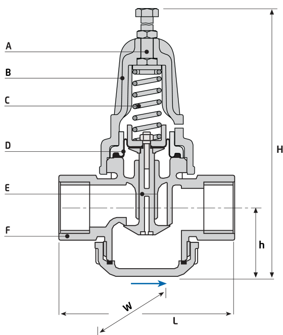
1-PRV Sezione trasversale
