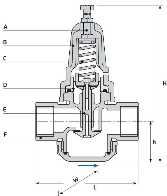
1-PRV-05 Sezione trasversale
