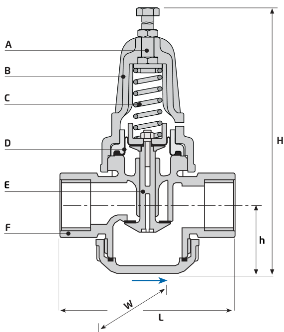
1-PRV-05 剖面图 - 法兰连接
