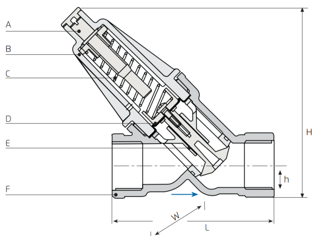
0.75-PRV Sezione trasversale
