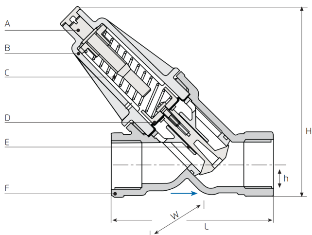
0.75-PRV 剖面图 - 法兰连接
