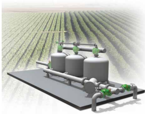
[1] BERMAD IR-430-50-2W-R 型阀门在收到压力下降指令时开启，维持过滤器反冲洗压力
