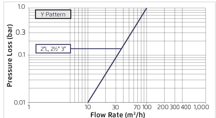
Círculo de 2 vías "Pérdida de carga añadida" (para "V" por debajo de 2 m/s): 0,3 bar
