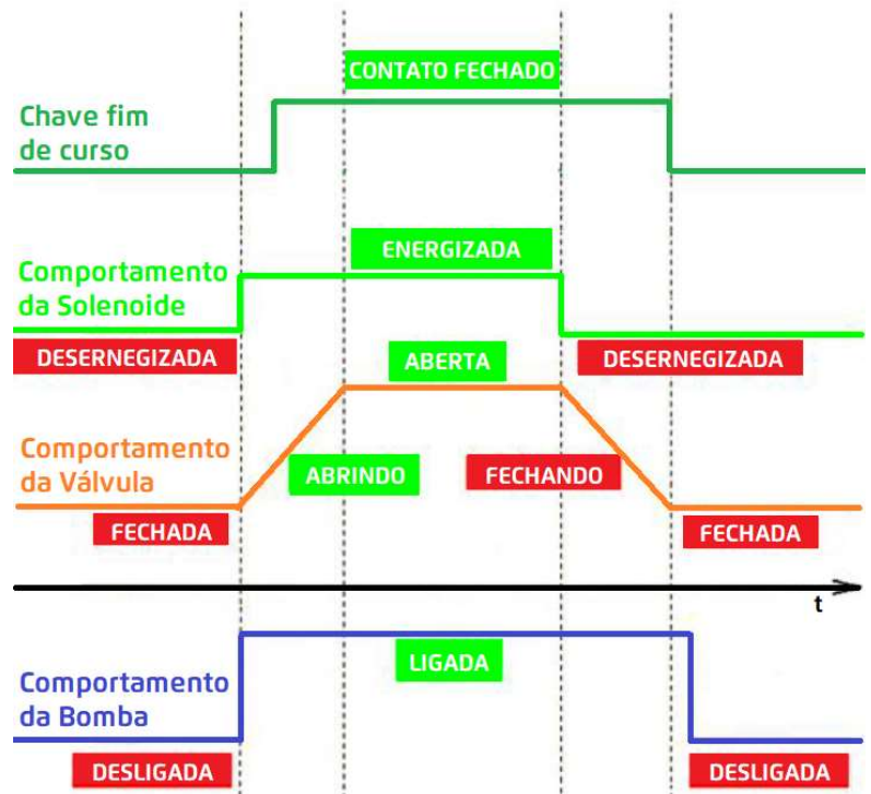
Comportamento da Partida de Bomba
